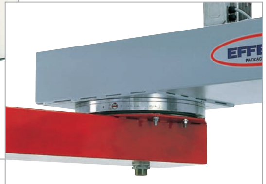
Gruppo rotazione su ralla a sfere comandata tramite motore autofrenante
